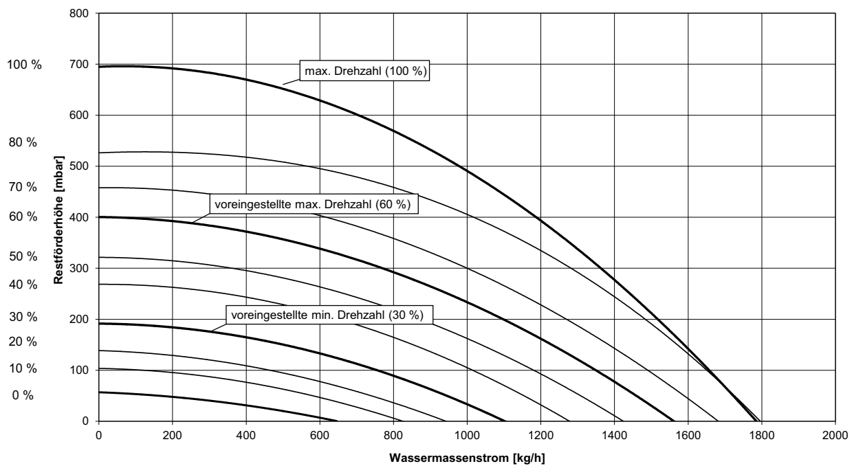
Abb. 9: Restförderhöhe BBK EVO 20/22 i
