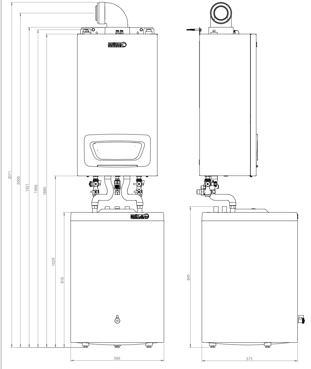
Abb. 10: WGB EVO 15–38 i mit BS 120 C
