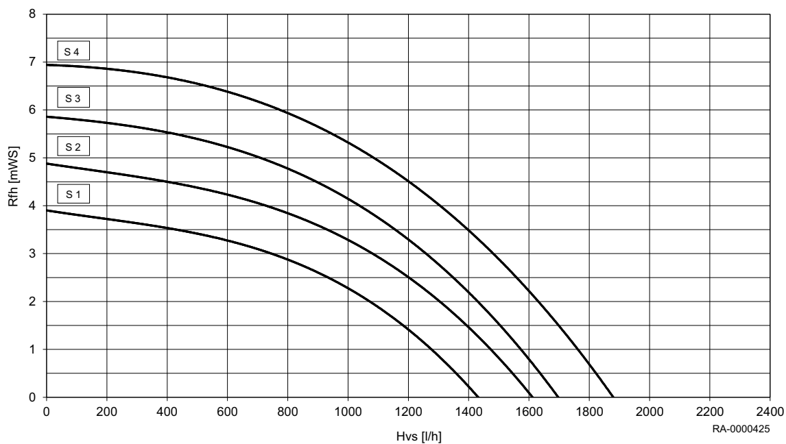
Abb. 19: Restförderhöhe WGB-M EVO 20 i für Mischerheizkreis (Einstellung Stufe 1–4)
